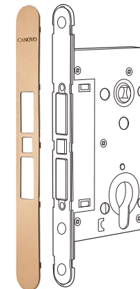
J5572-E Double magnetic mortise lock 双磁锁体
