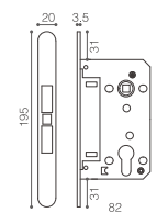
J5572-E Double magnetic mortise lock 双磁锁体
