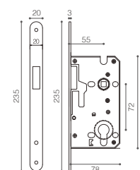
J5572-M Magnetic Mortise Lock 磁力锁体
